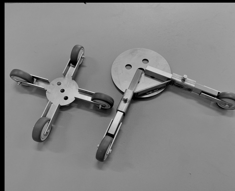
FAHRWERK FÜR PACKER 200/500 und 300/1000
